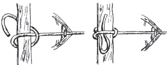
шлюпочный узел
